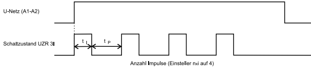
Taktgeber mit Impulsbeginn (B1 offen)
