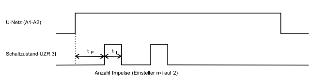
Taktgeber mit Pausenbeginn (B1 - A1 gebrückt)
